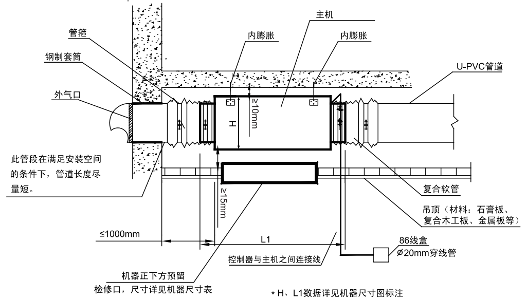
○ 安装大样图
