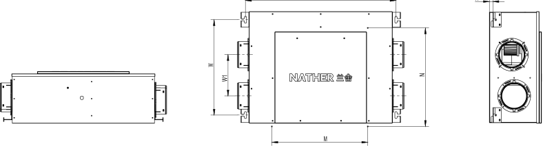
GA-2a安装尺寸图
